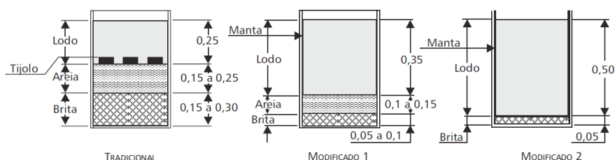
Figura 2: Etapas de desenvolvimento do Leito de Drenagem (LD) com valores em metros.
