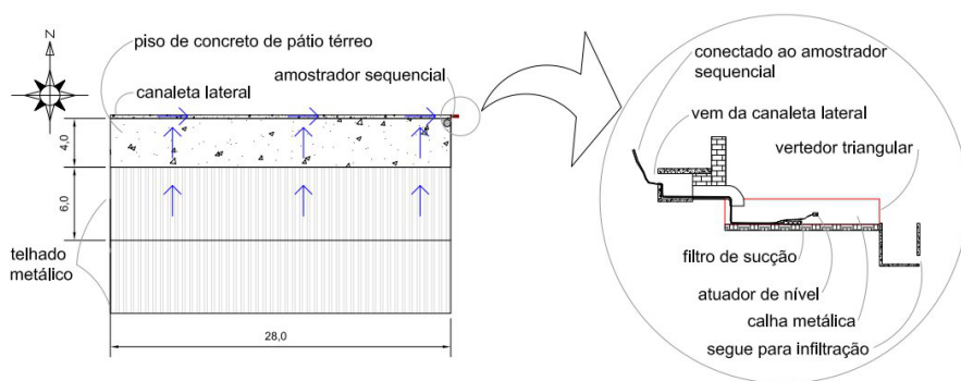
Figura 1 – Planta do prédio do laboratório de polímeros biodegradáveis, com detalhamento da calha metálica.
