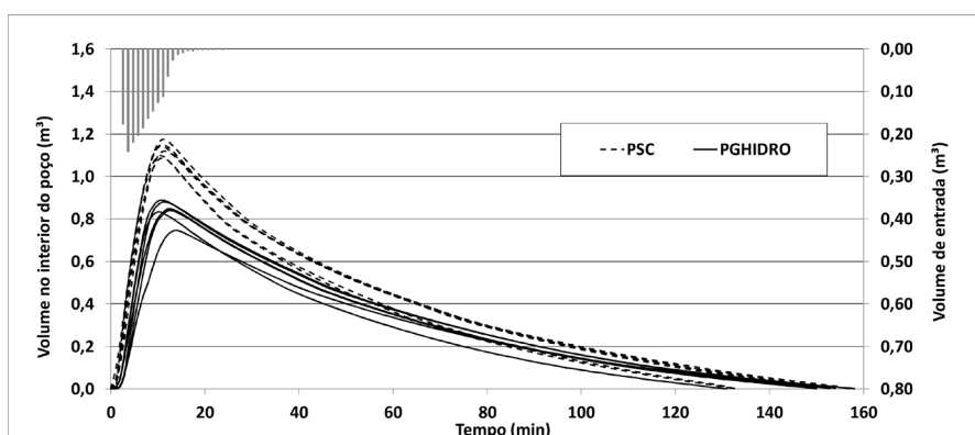
Figura 3: Volumes no interior dos poços de infiltração sob o mesmo volume de entrada em do função tempo.
