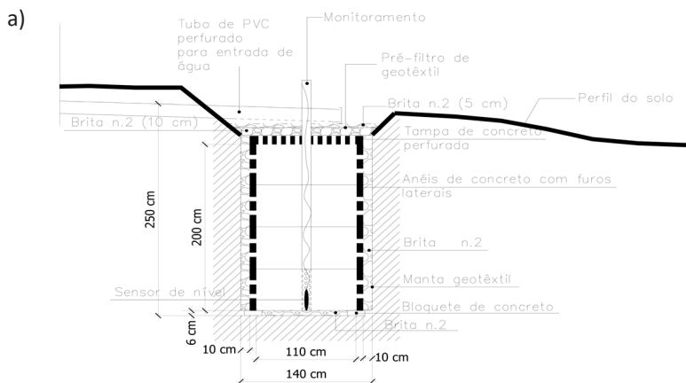
Figura 1: Cortes do poço PGHIDRO (a) e do poço PSC (b)
