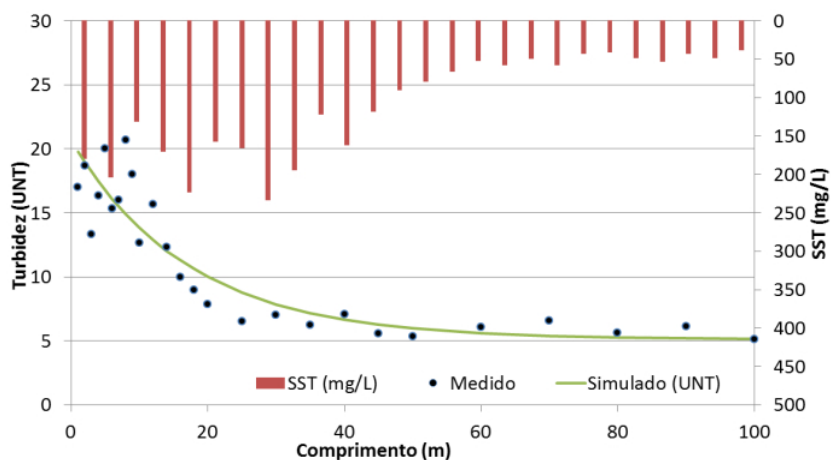
Figura 4 – Concentração residuais remanescentes de material particulado medidas e simuladas com relação à posição. Resultados em unidades de turbidez no eixo principal das ordenadas e em sólidos suspensos totais no eixo secundário das ordenadas. Condições dos ensaios: C_0 de 195 \text{ mg} \cdot \text{L}^{-1} ; q de 0,15 \text{ m}^3/\text{s} \cdot \text{m}^2 ; t_b de 25 min; t_b/t_T de 2,4.
