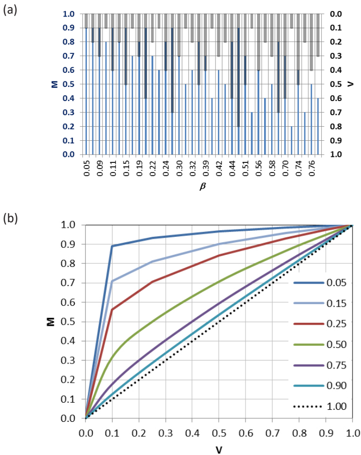
Figura 2 – (a) Frações de massa transportada (M) e de volume (V) para diversos valores do coeficiente \beta e (b) frações de massa transportada (M) em função da fração volume (V) também para diversos valores de do coeficiente \beta para 0 < \beta < 1 .
