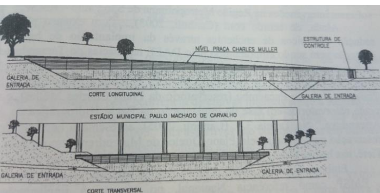
Bacia de detenção subterrânea
